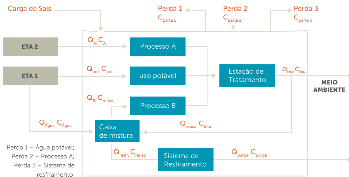
Figura 3.6 Avaliação da concentração de sais em um sistema de reúso de água
