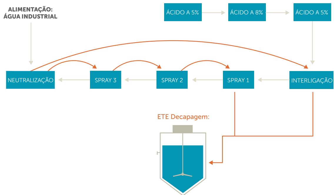
Figura 4.1 Esquema do processo de decapagem
