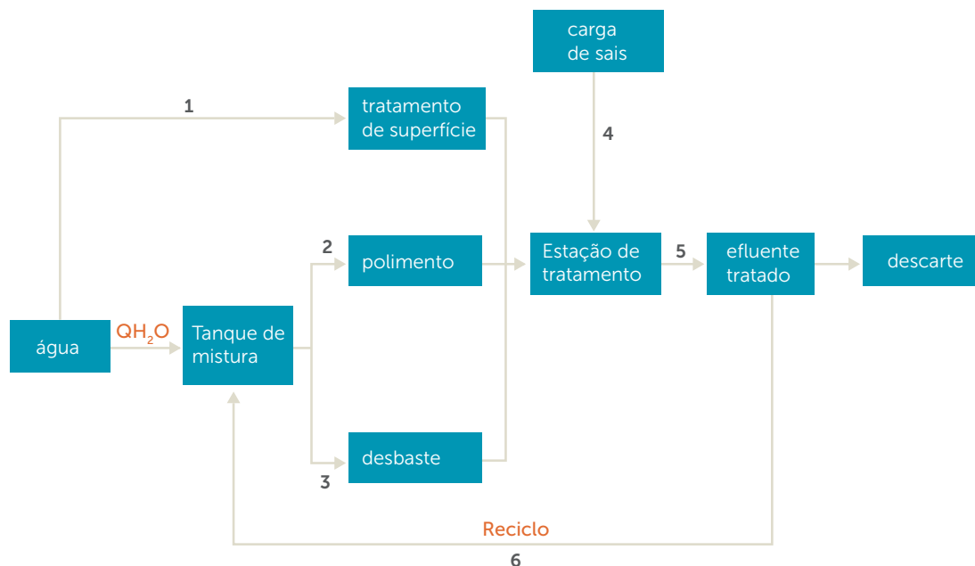
Figura 4.3 Esquema do balanço de massa para determinação do reúso de água
