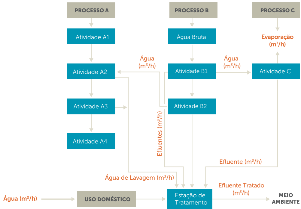
Figura 3.2 Fluxos de água e efluentes em uma unidade industrial (Mierzwa e Hespagnol, 2005).
