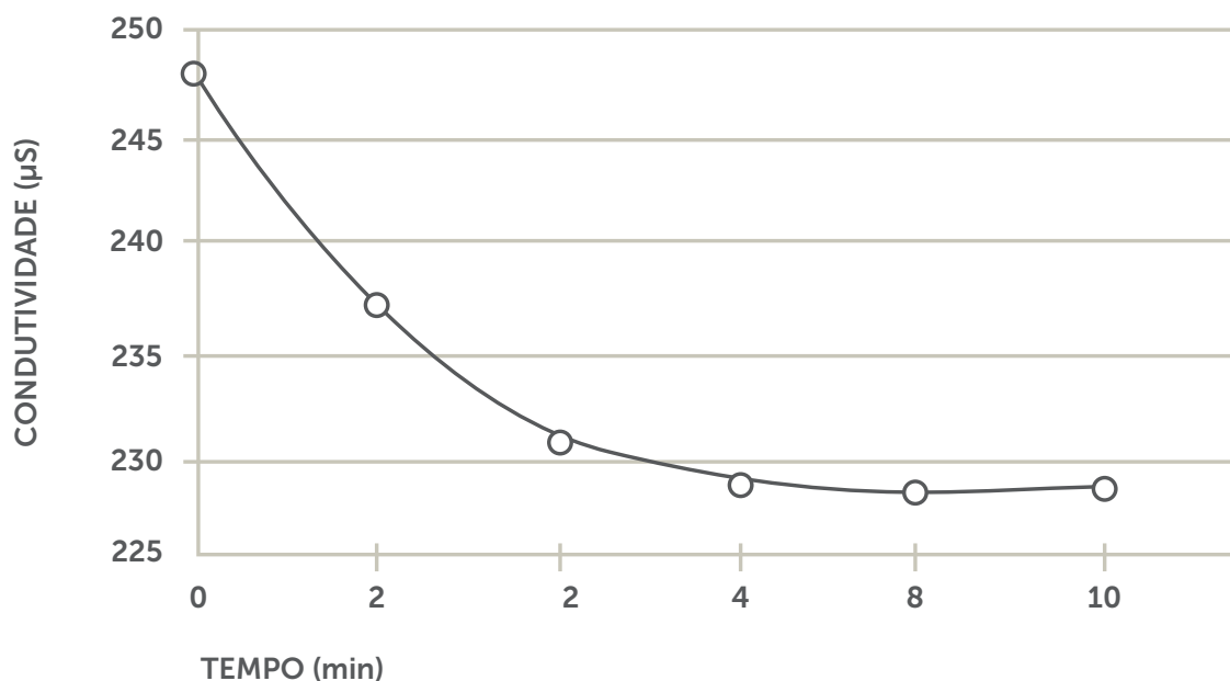
Figura 3.5 Curva referente ao decaimento da condutividade em função do tempo de lavagem
