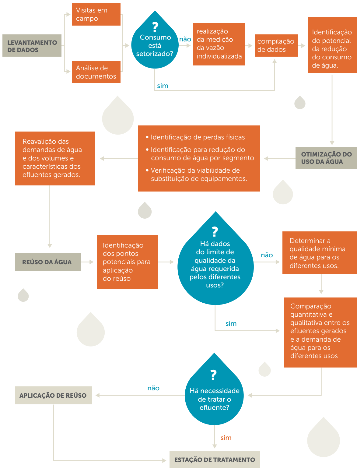
Figura 3.1 Diagrama para desenvolvimento do PCRA
